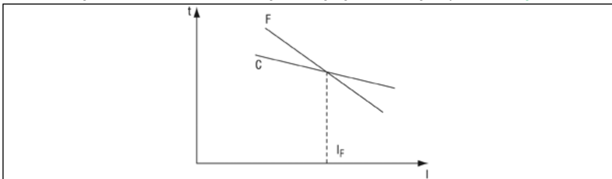
Figuur 5.43. Keuze van de beschermingsinrichting tegen kortsluitingen bij smeltzekeringen
