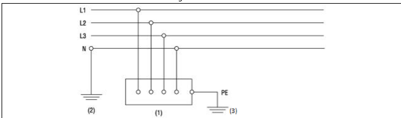
Figuur 3.2. TT-net
