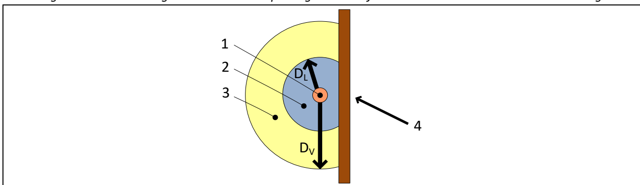
Figuur 2.29. Voorstelling van de zone onder spanning en de nabijheidszone met isolerende beschermrichting
