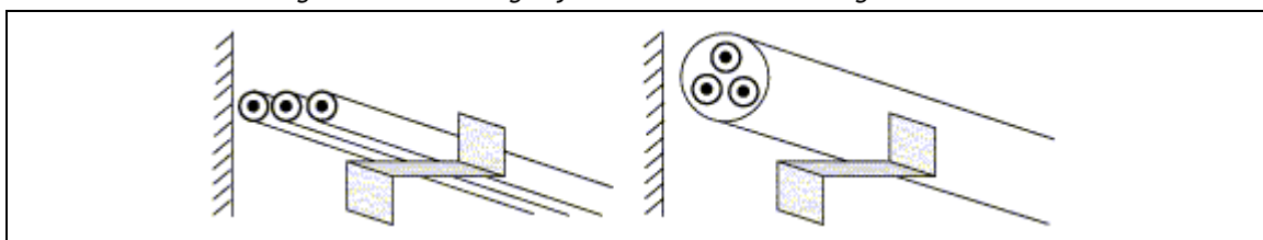
Figuur 5.27. Plaatsingswijzen van elektrische leidingen – Haken
