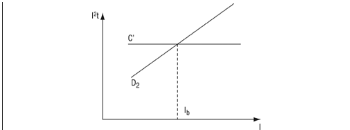
Figuur 5.45. Keuze van de beschermingsinrichting tegen kortsluitingen bij vermogensschakelaars (veronderstelde kortsluitstroom)
