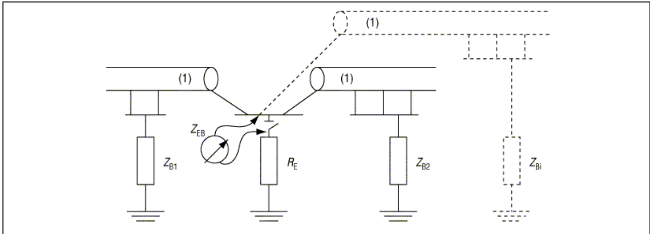
Figuur 2.16. Lusimpedantie van een aardverbinding Z_{EB}
