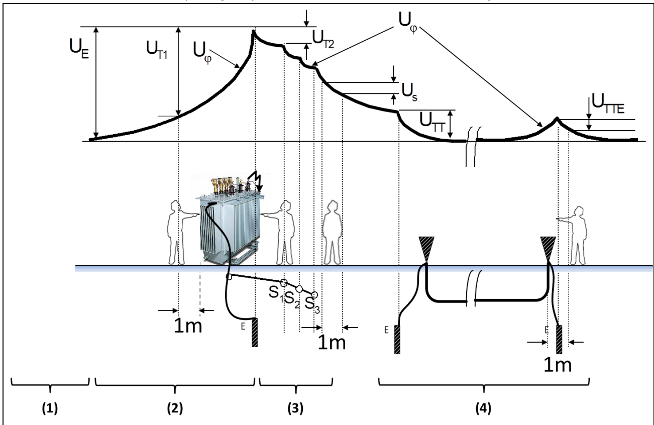
Figuur 2.12. Voorbeeld van verandering van aardbodemsparing en van spanningen bij het vloeien van stroom in de aardverbindingen
