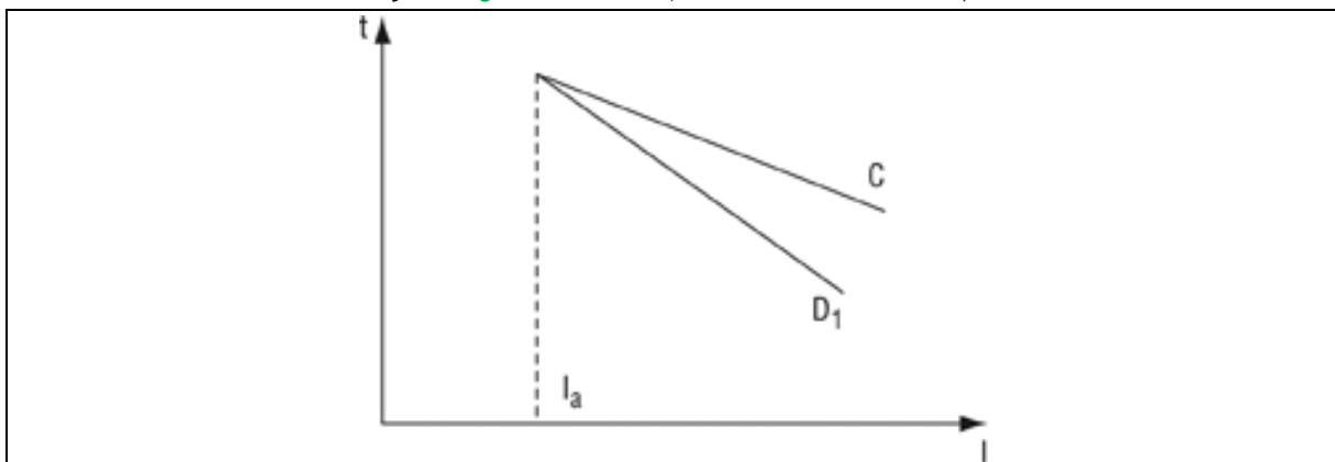
Figuur 5.44. Keuze van de beschermingsinrichting tegen kortsluitingen bij vermogensschakelaars (minimale kortsluitstroom)
